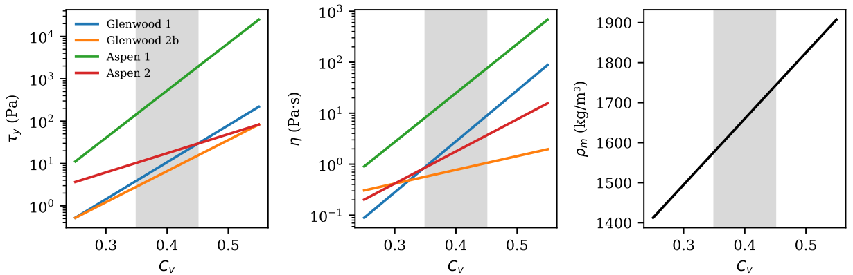
Figura 3: Propiedades de la mezcla según la concentración volumétrica de sólidos C_v para las muestras ensayadas: esfuerzo de fluencia \tau_y , viscosidad \eta y densidad \rho_m . La franja gris indica el rango usado (0,35–0,45).
