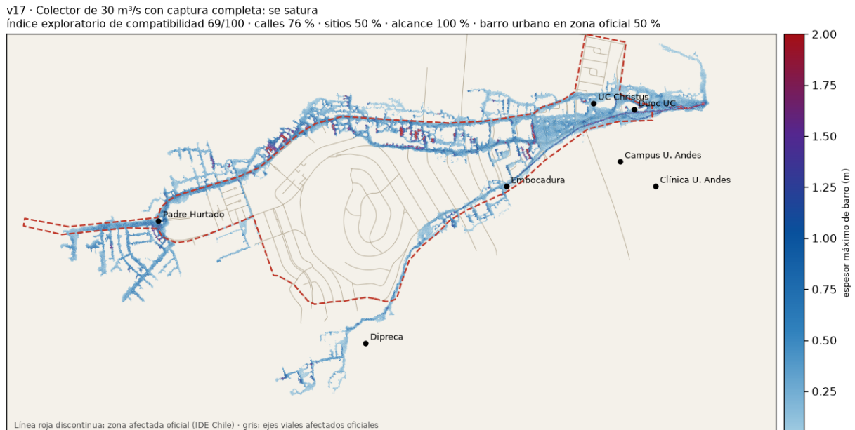
Figura 12: Ficha v17: Colector de 30 m 3 /s con captura completa: se satura.
