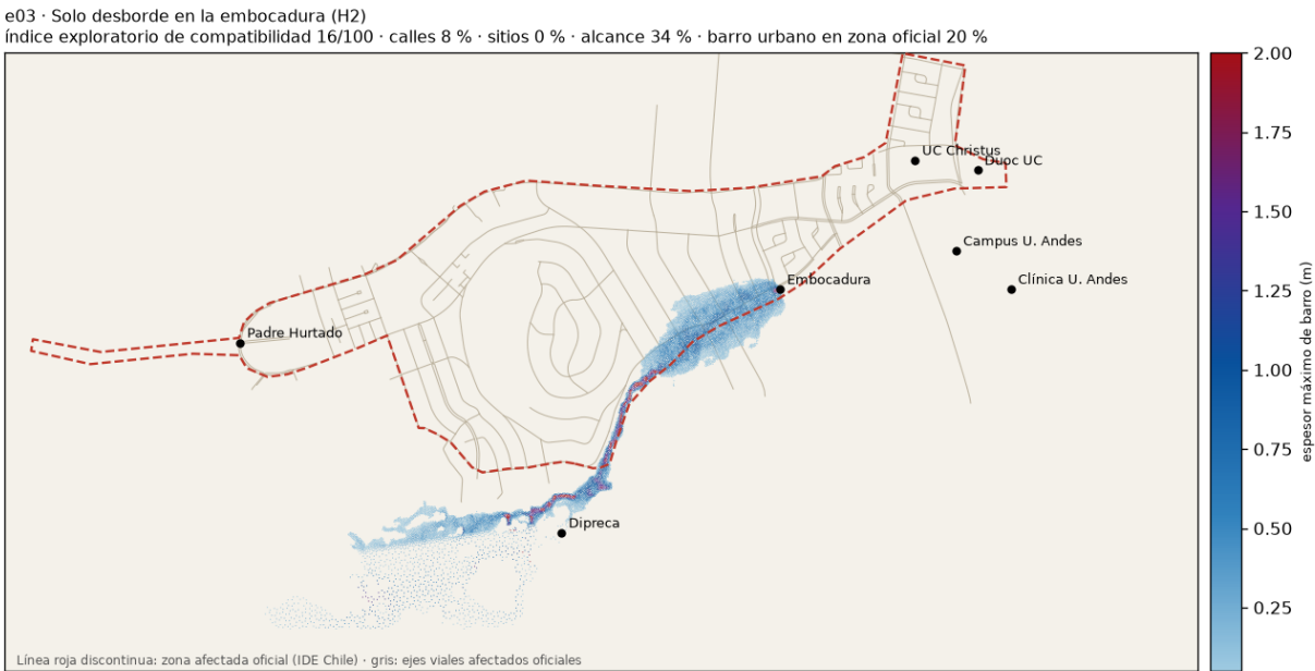
Figura 18: Ficha e03: Solo desborde en la embocadura (H2).
