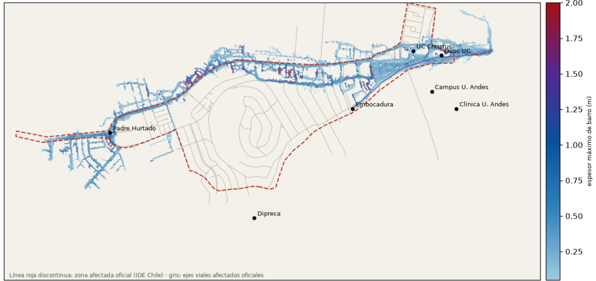
Figura 13: Ficha v10: Escenario hipotético: capacidad del colector fijada en 100 m³/s.
