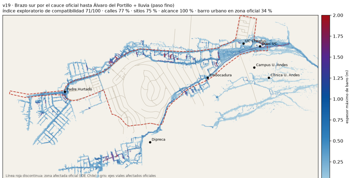
Figura 11: Ficha v19: Brazo sur por el cauce oficial hasta Álvaro del Portillo + lluvia (paso fino).
